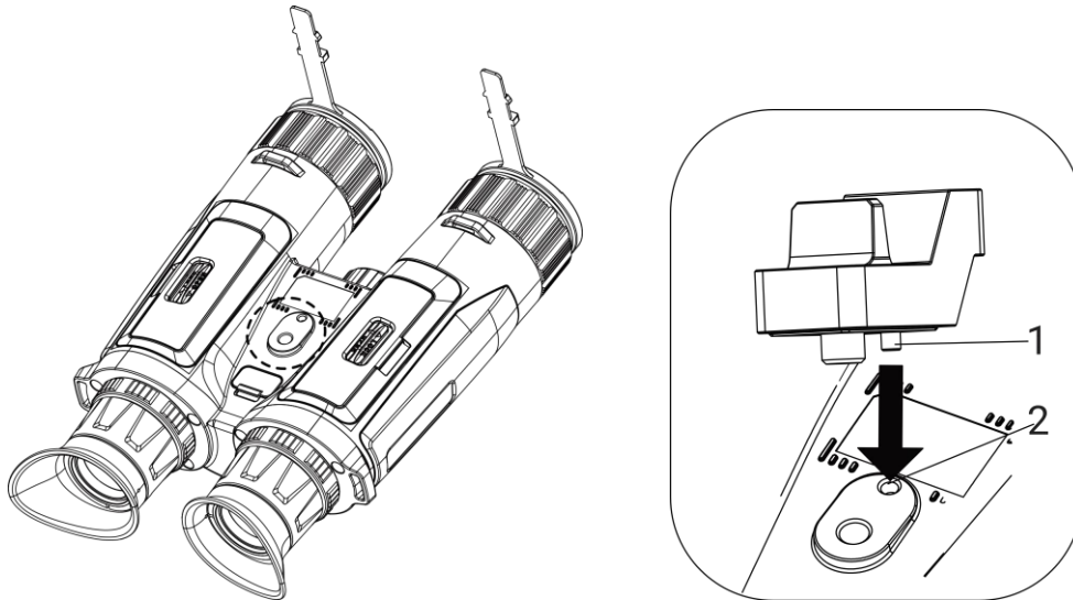
Abbildung 2-8 Den Führungsstift einsetzen
